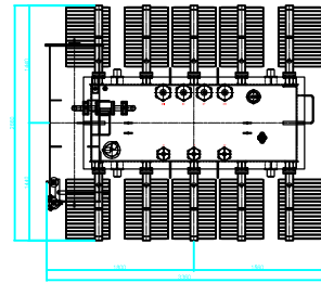
Detail bovenaanzicht transformator
